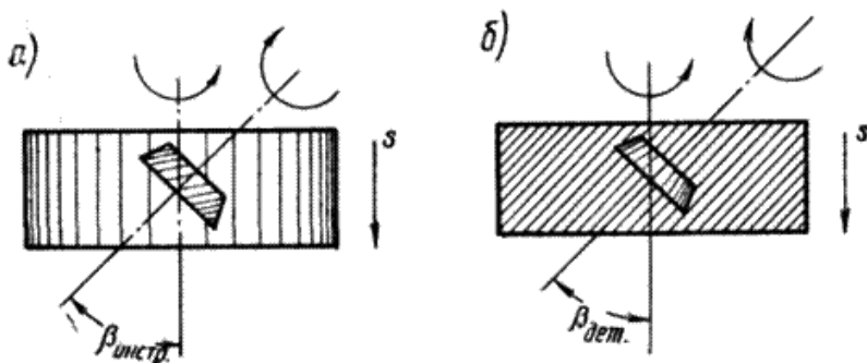
Рис. 1. Схемы установки и кинематика обработки цилиндрических зубчатых колес:
